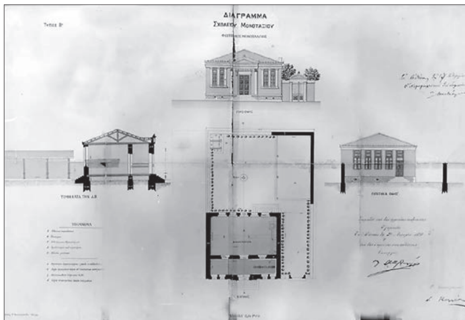
Δ. Καλλιὰς, Διάγραμμα Μονοταξίου Δημοτικού Σχολείου, Τύπος Β', 1898, ἀπό: Μάρω Καρδαμίτση-Ἀδάμη, ὁ Δ. Καλλιὰς καὶ τὸ Σχολικὸ Κτίριο, Ἐθνικὸ Μετσόβιο Πολυτεχνεῖο, Ἀθήνα 1986.
